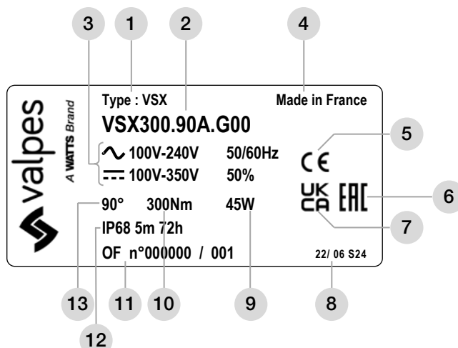
Placa de identificación del actuador (exterior - Carcasa)
